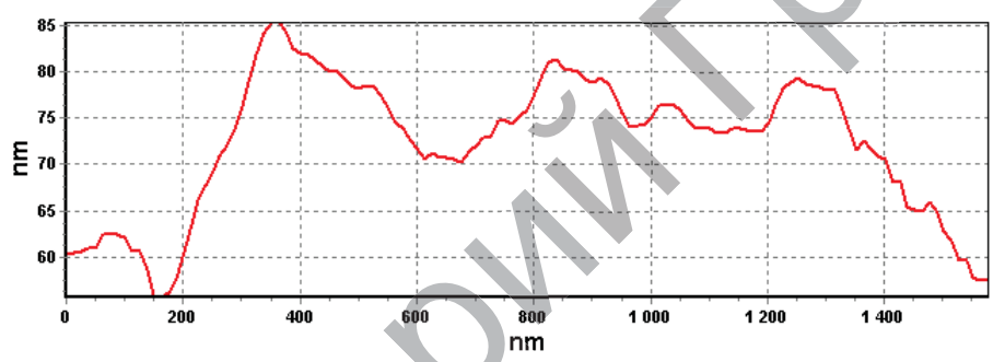
Рисунок 4 – Профилограмма, вдоль линии, на рисунке 3,б
