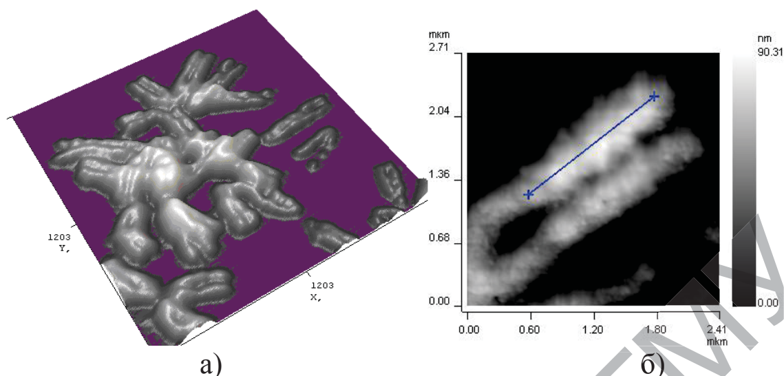
Рисунок 3 – АСМ- изображение: а) 3D, б) 2D с линией профиля
