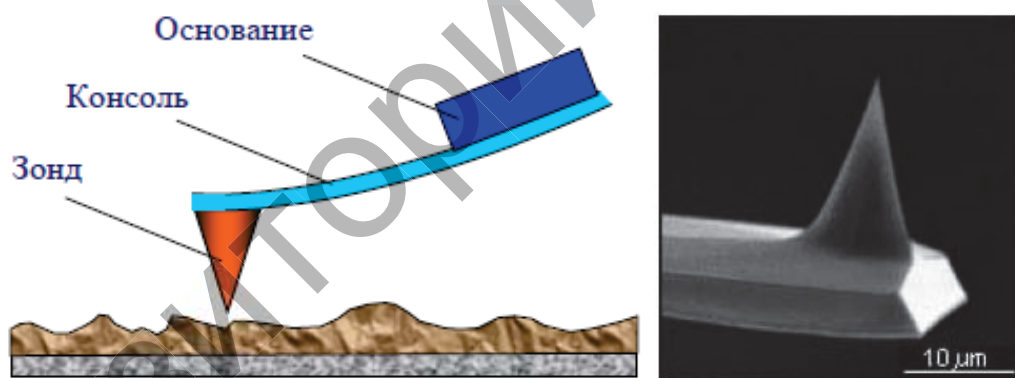
Рисунок 1 – Схематическое изображение АСМ и снимок зонда [5]
