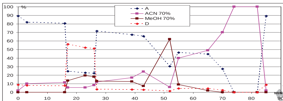
Рисунок 2 – Профиль градиентного элюирования для определения свободных аминокислот
